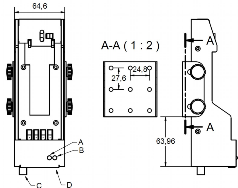
Schemazeichnung WTC1904
