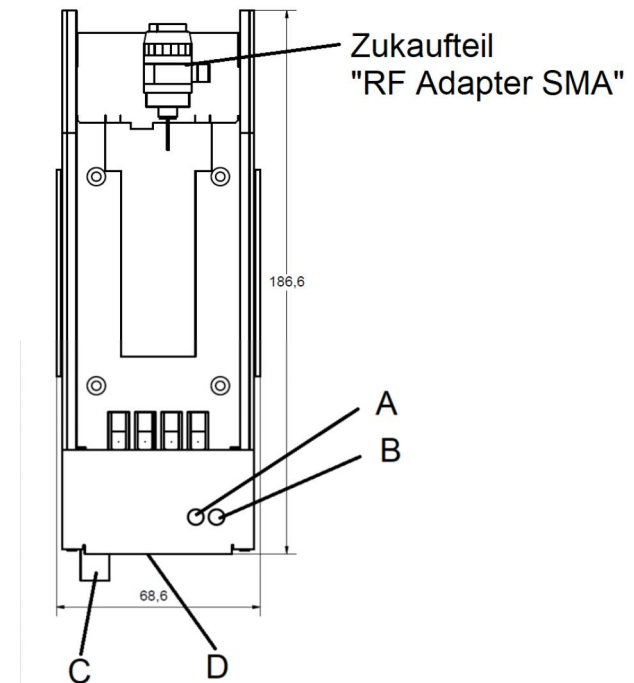
Schemazeichnung WTC679
