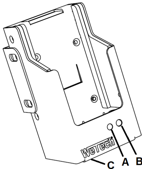
Schemazeichnung WTC681
