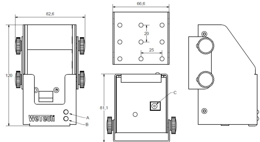
Schemazeichnung WTC695
